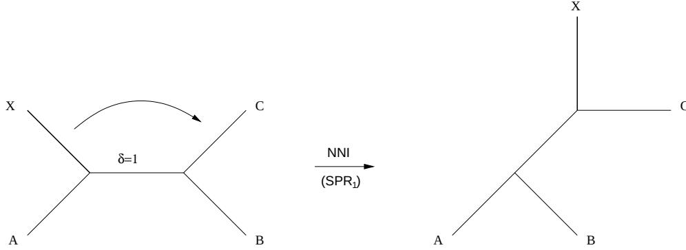
FIGURE 5.2 – NNI et le voisinage paramétrique : NNI correspond au cas où d = 1
