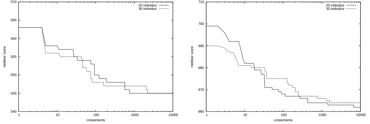
FIGURE 6.5 – Influence de la taille de la population
