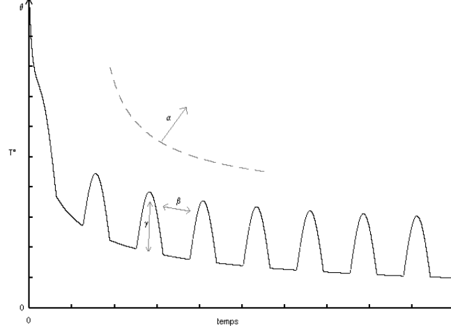
FIGURE 4.3 – Schéma de réduction non-monotone de la température
