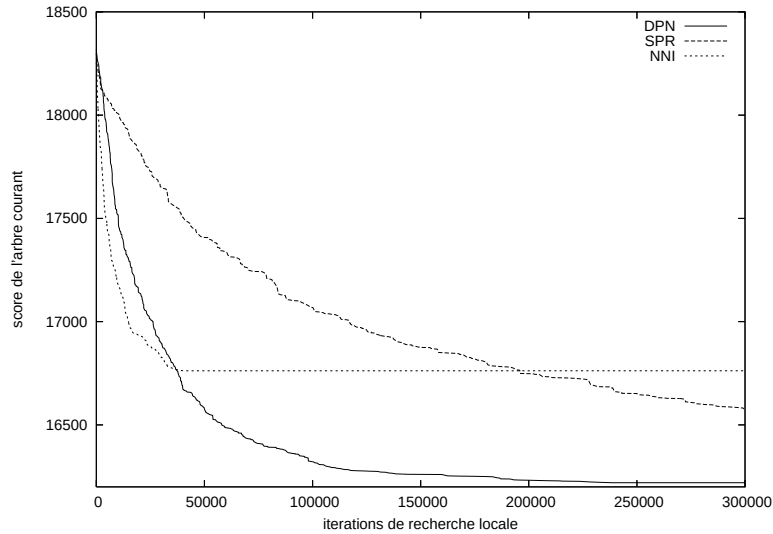
FIGURE 5.9 – Évolution du score de la solution courante depuis une solution intermédiaire construite par UPGMA (instance zilla)
