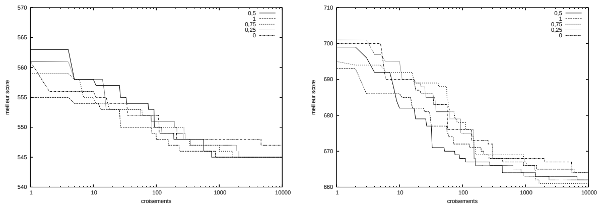
FIGURE 6.7 – Influence de la définition de la métrique \delta dans le croisement
