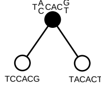
FIGURE 2.3 – Séquence de parcimonie
