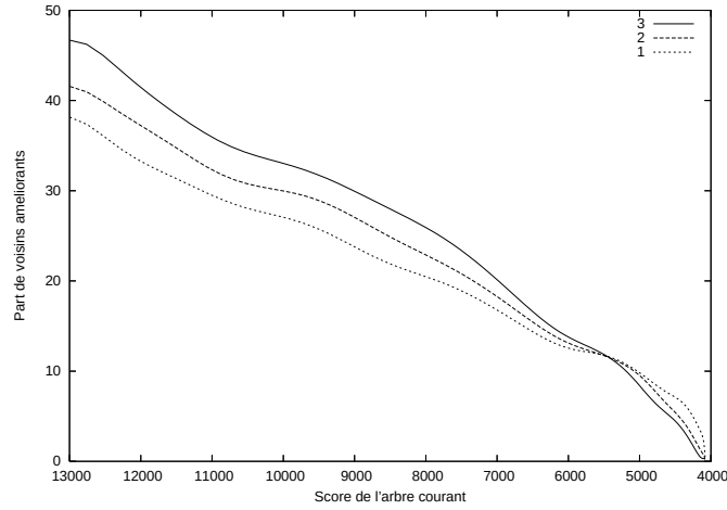
FIGURE 5.6 – Évolution de la proportion de voisins améliorants en fonction du score des solutions, pour une distance \delta donnée (3, 2, 1)
