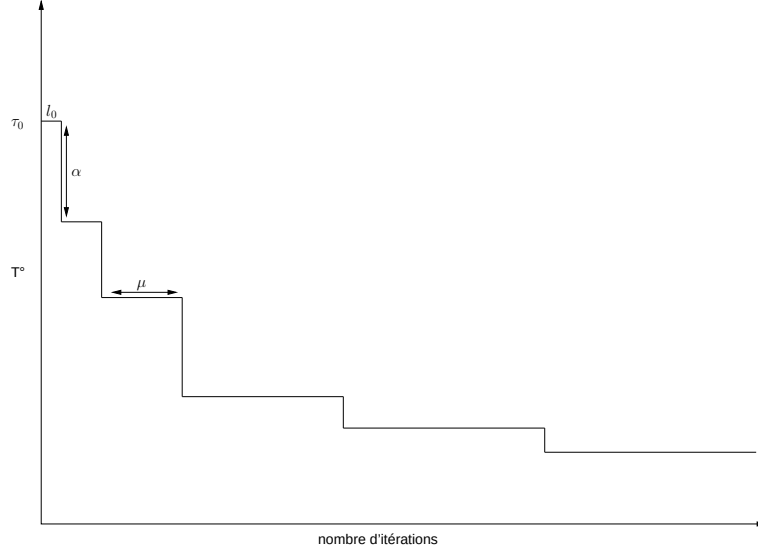
FIGURE 4.2 – Schéma de réduction de la température par paliers
