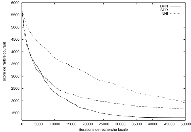
FIGURE 5.7 – Évolution des scores des arbres courants pour les descentes SPR, NNI et DPN sur l'instance 300-100-5 depuis un arbre aléatoire
