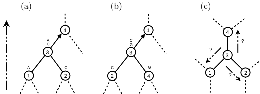
FIGURE 2.8 – La présence d'une racine entraîne une hiérarchisation des nœuds
