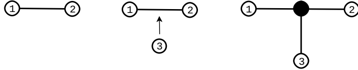
FIGURE 1.2 – Arbres triviaux à deux ou trois taxons
