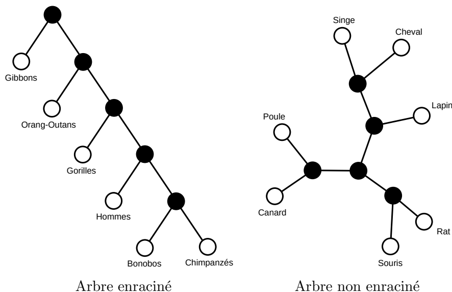
FIGURE 1.1 – Exemples d'arbres phylogénétiques enracinés ou non
