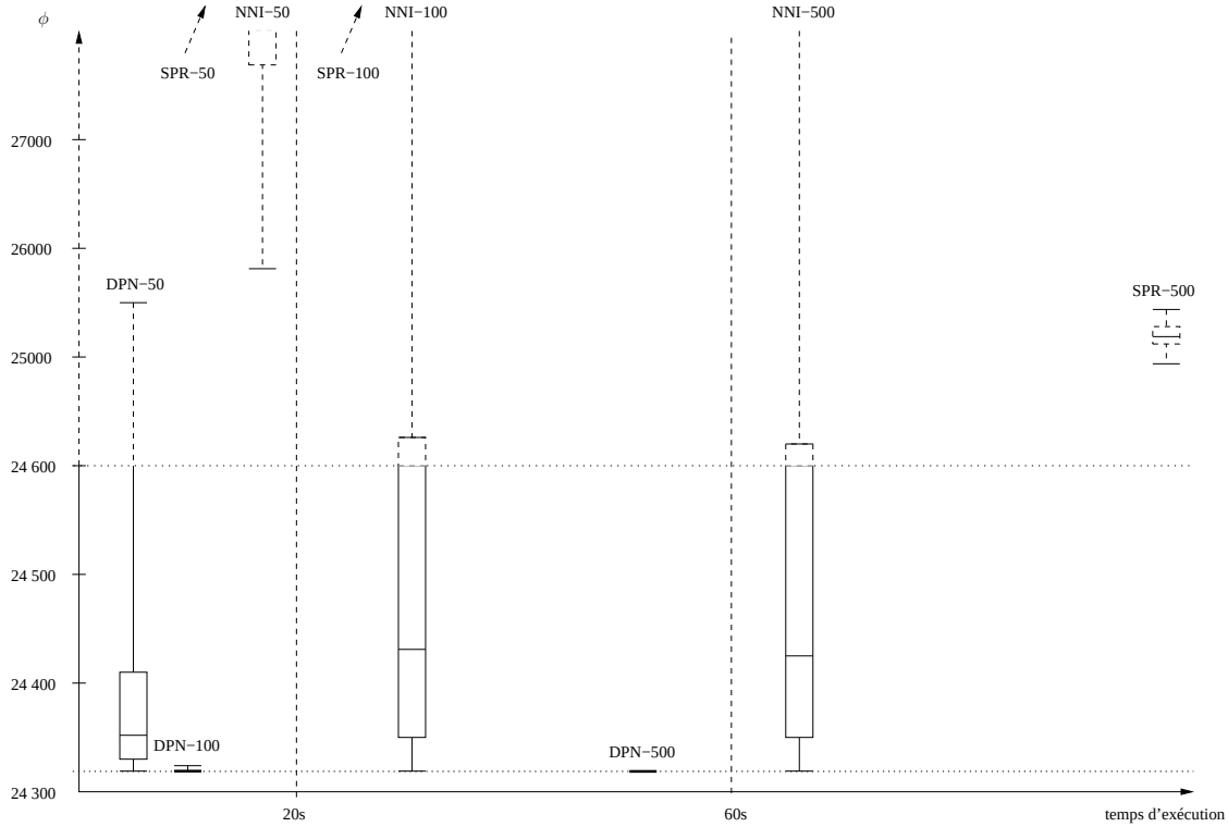
FIGURE 5.8 – Performances comparées sur l'ensemble des exécutions (instance 500–1000–5)
