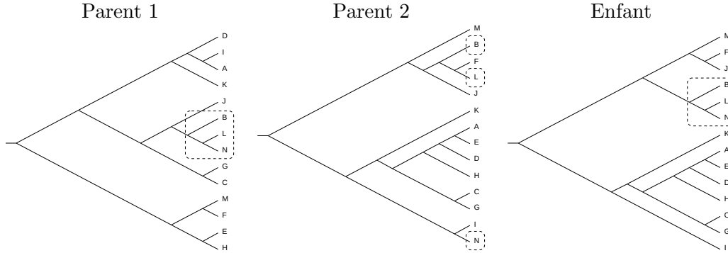
FIGURE 6.2 – Résultat d'un croisement d'arbres classique
