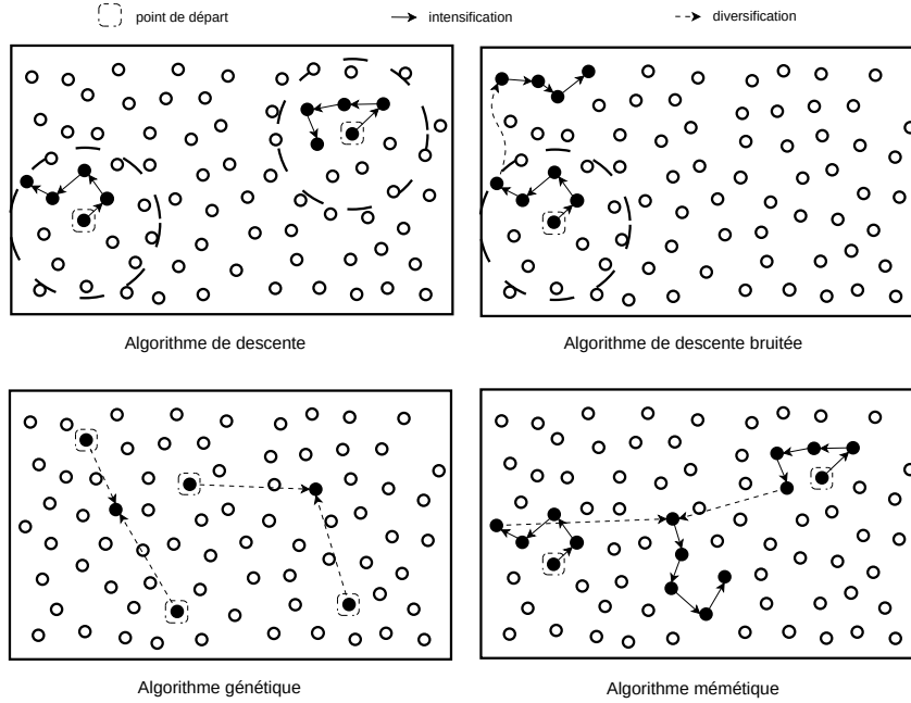
FIGURE 6.1 – Fonctionnement d'un algorithme mémétique
