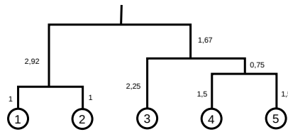
FIGURE 1.4 – Exemple de dendrogramme obtenu par l'algorithme UPGMA
