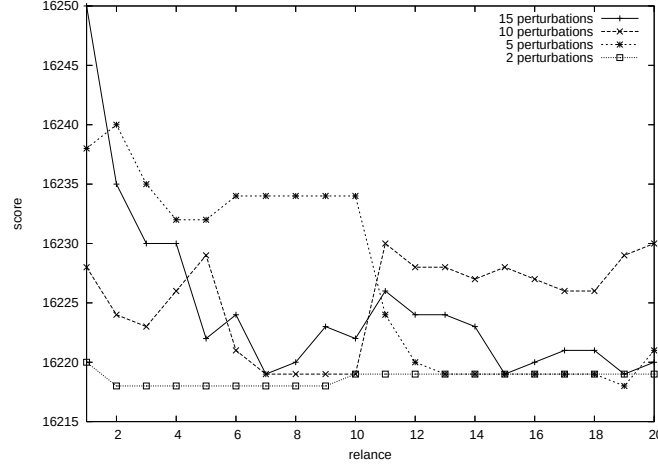
FIGURE 4.1 – Évolution des recherches locales itérées
