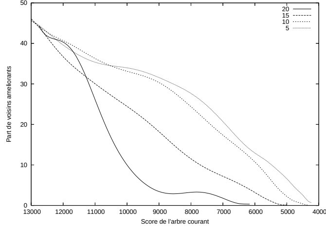
FIGURE 5.5 – Évolution de la proportion de voisins améliorants en fonction du score des solutions, pour une distance \delta donnée (20, 15, 10, 5)
