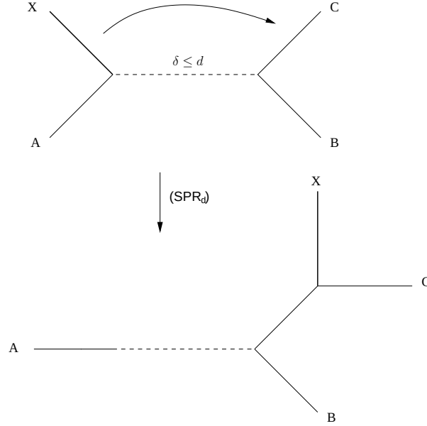
FIGURE 5.1 – SPR et le voisinage paramétrique : SPR correspond au cas où d = \infty
