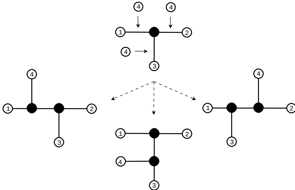
FIGURE 1.3 – Différents placements possibles pour un quatrième taxon
