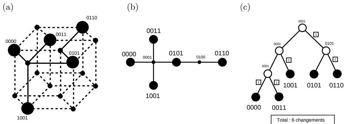
FIGURE 2.6 – Problème de Steiner dans un hypercube de dimension 4
