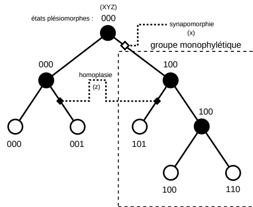
FIGURE 1.5 – Constitution d'un groupe monophylétique
