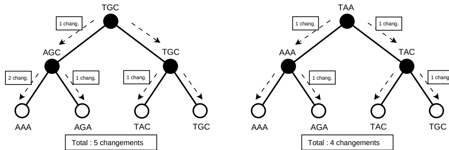
FIGURE 2.2 – Différentes séquences hypothétiques pour un même arbre
