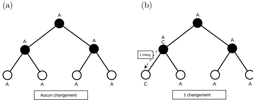
FIGURE 2.7 – Scores de parcimonie constants sur les sites non informatifs
