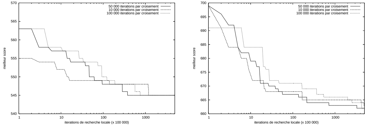
FIGURE 6.6 – Influence de la longueur de la recherche locale
