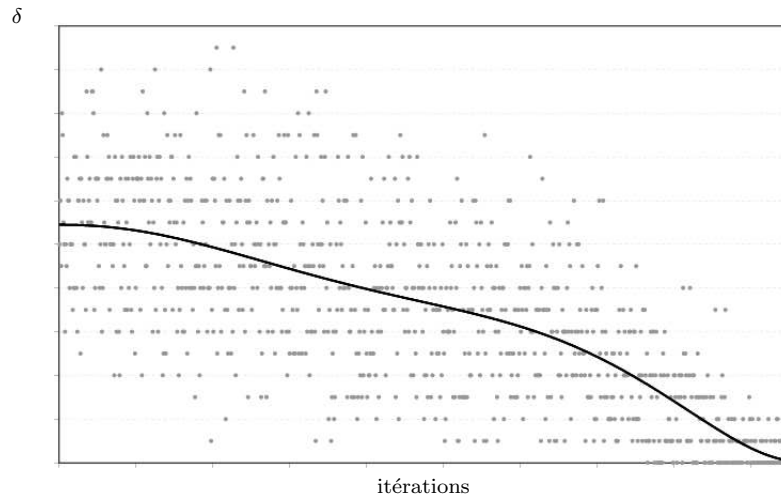
FIGURE 5.3 – Évolution de la distance \delta entre des arbres et leurs meilleurs voisins SPR, en fonction du nombre d'itérations.
