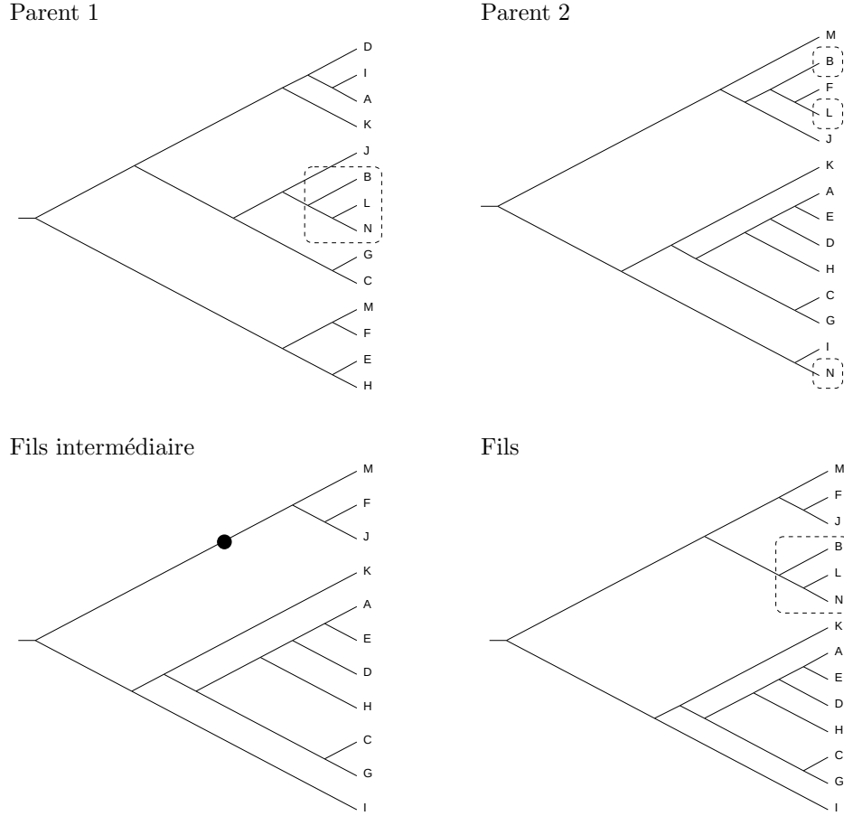
FIGURE 3.5 – Exemple de croisement d’arbres couramment utilisé
