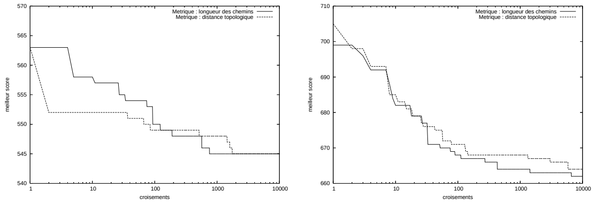
FIGURE 6.6 – Influence de la longueur de la recherche locale
